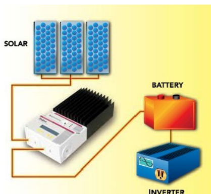
1. Kontroler ładowania
