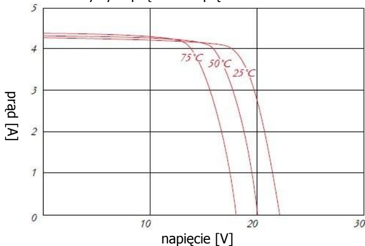
Charakterystyka prądowo-napięciowa
