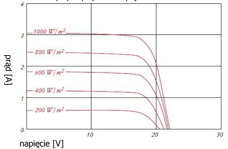
Charakterystyka prądowo-napięciowa
