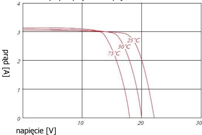
Charakterystyka prądowo-napięciowa
