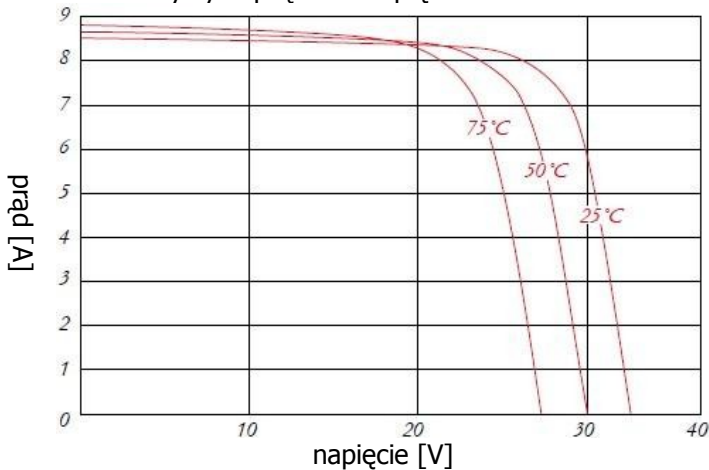
Charakterystyka prądowo-napięciowa
